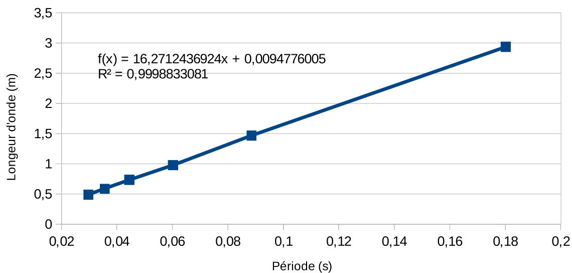
Longueur d'onde en fonction de la période pour 140g
