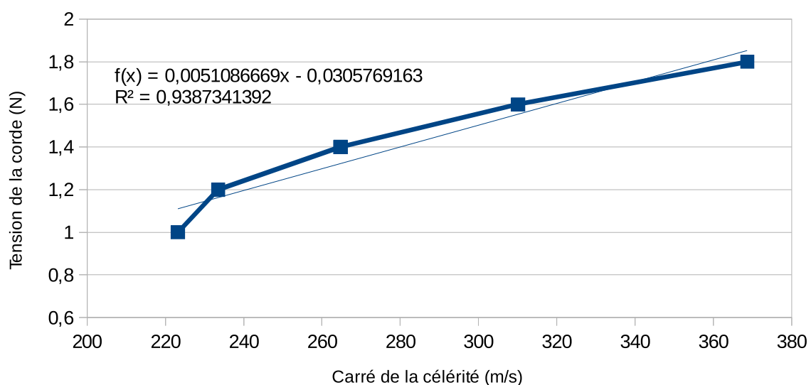
Tension de la corde en fonction du carré de la célérité
