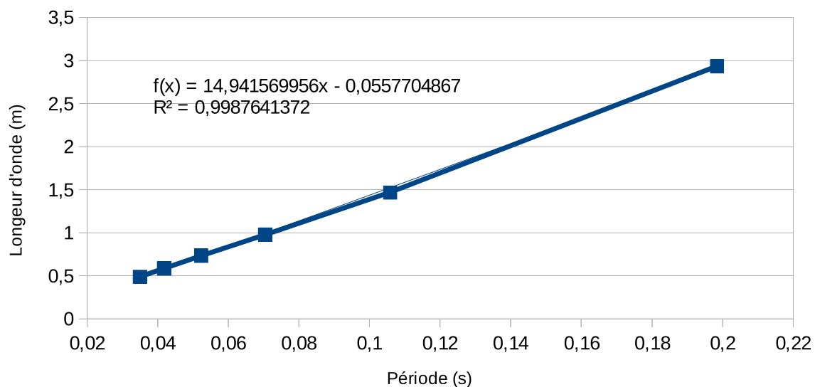
Longueur d'onde en fonction de la période pour 100g
