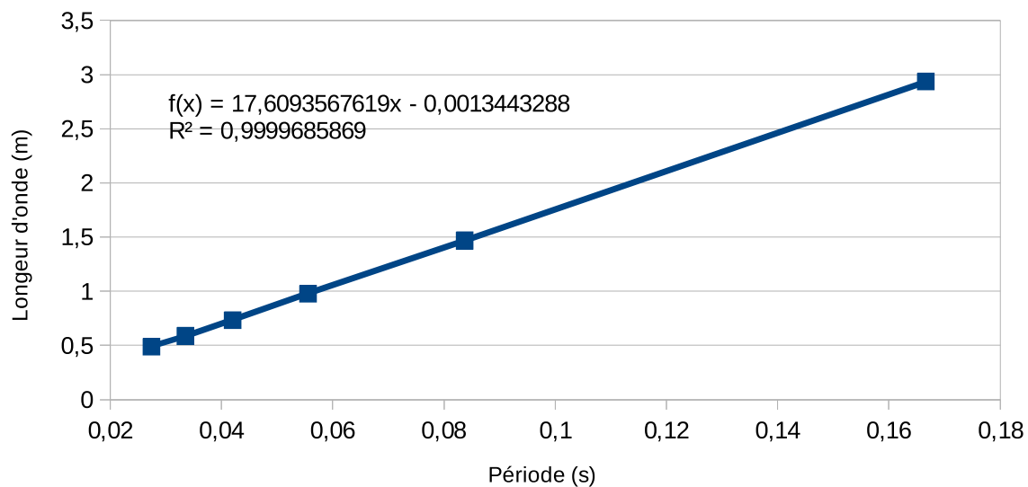
Longueur d'onde en fonction de la période pour 160g
