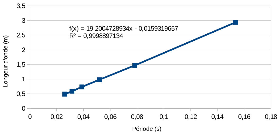
Longueur d'onde en fonction de la période pour 180g
